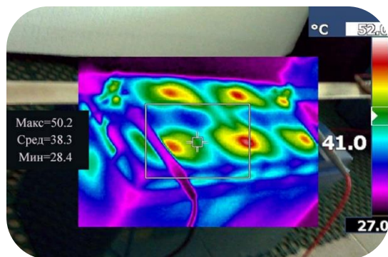
Рост температуры клемм обычного аккумулятора в конце разряда
