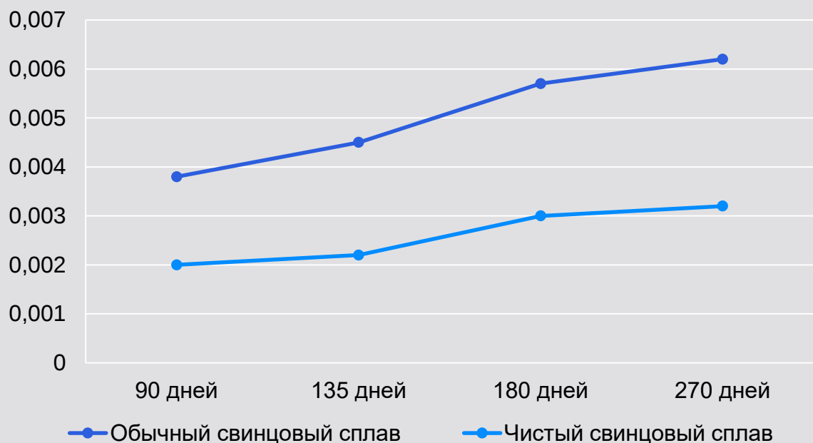
Сравнение месячной коррозии пластин, мм
