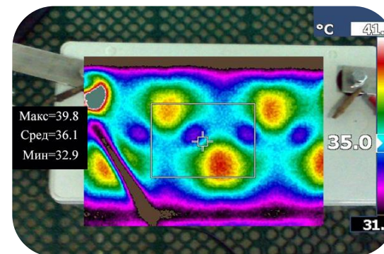
Рост температуры клемм высокоэффективного аккумулятора в конце разряда
